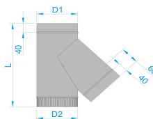
Трійник з нержавіючої сталі товщиною 0,5мм
