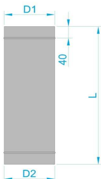
Труба з нержавіючої сталі товщиною 0,5мм
