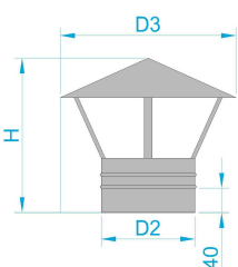
Дашок з нержавіючої сталі товщиною 0,5мм
