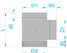
Трійник з нержавіючої сталі товщиною 0,8мм
