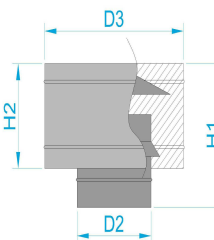
Дефлектор з нержавіючої сталі товщиною 0,8мм
