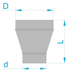
Прехідник з нержавіючої сталі товщиною 0,8мм
