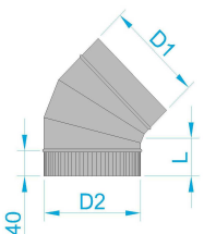
Коліно з нержавіючої сталі товщиною 0,5мм
